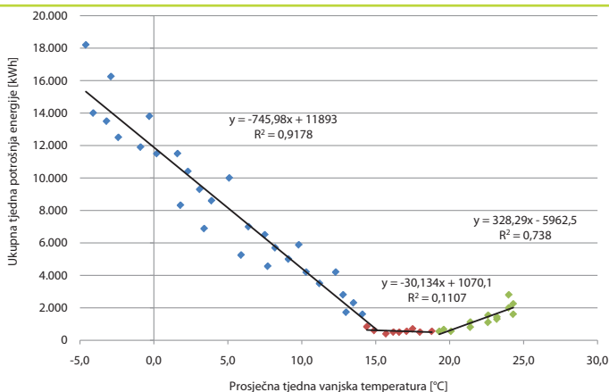
Slika P-14: Primjer E-T krivulje ukupne energije sa silaznim zimskim razdobljem, prijelaznim razdobljem i uzlaznim ljetnim razdobljem
