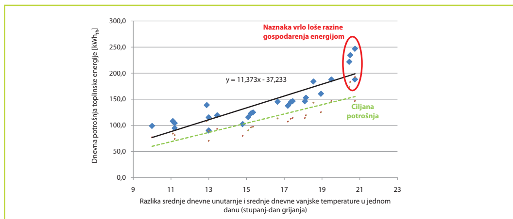
Slika 6-6: Primjer prikaza dnevne potrošnje toplinske energije u ovisnosti o stupanj-danu grijanja regresijskom metodom
