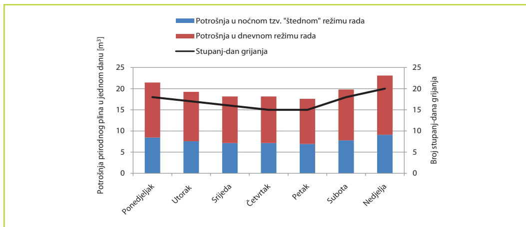
Slika 6-2: Primjer prikaza dnevne potrošnje prirodnog plina po funkcijskim periodima i stupanj-dana grijanja u odabranom tjednu
