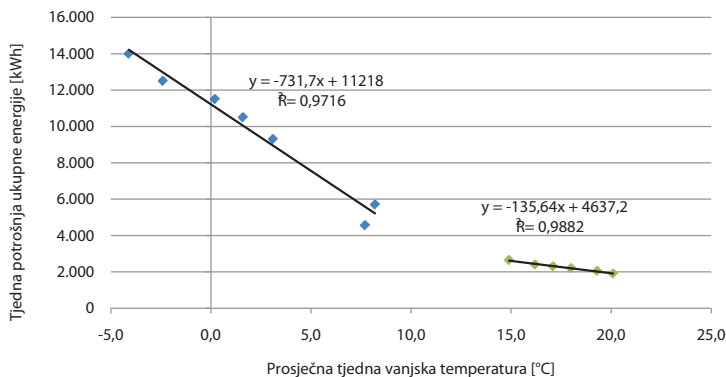
Slika 5-6: Primjer bazne E-T krivulje
