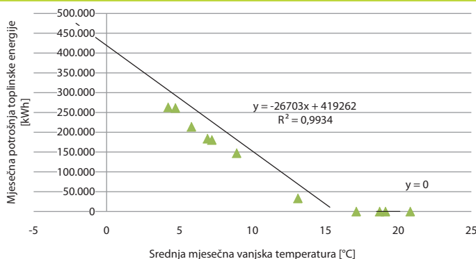
Slika 6-12: Mjesečna potrošnja toplinske energije u ovisnosti o vanjskoj temperaturi u 2008. godini uz naznačenu baznu potrošnju
