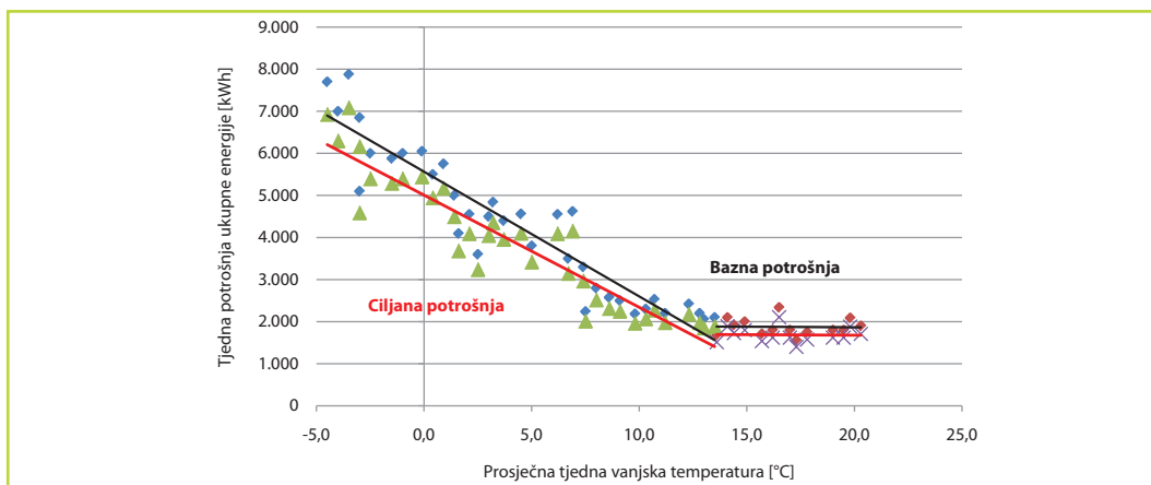
Slika 5-7: Primjer prikaza ciljane E-T krivulje odabirom smanjenja potrošnje u iznosu od 10%
