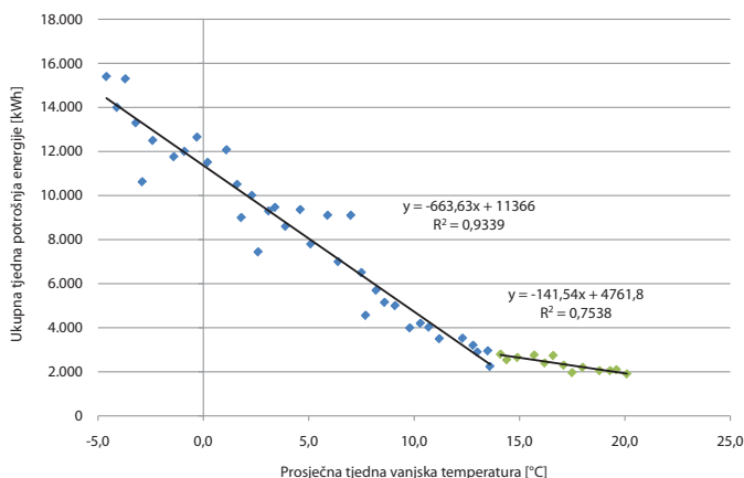
Slika P-11: Primjer E-T krivulje ukupne energije sa silaznim zimskim razdobljem i silaznim ljetnim razdobljem
