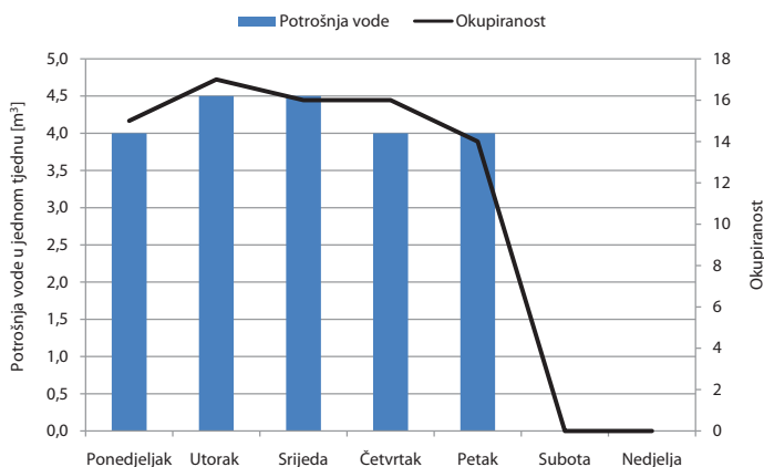
Slika 6-3: Primjer prikaza potrošnje vode i razine okupiranosti u odabranom tjednu
