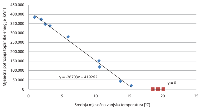
Slika 6-11: Mjesečna potrošnja toplinske energije u ovisnosti o vanjskoj temperaturi u baznoj 2007. godini
