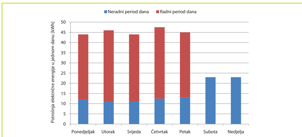
Slika 5-2: Primjer prikaza dnevne potrošnje električne energije u odabranom tjednu po funkcijskim periodima
