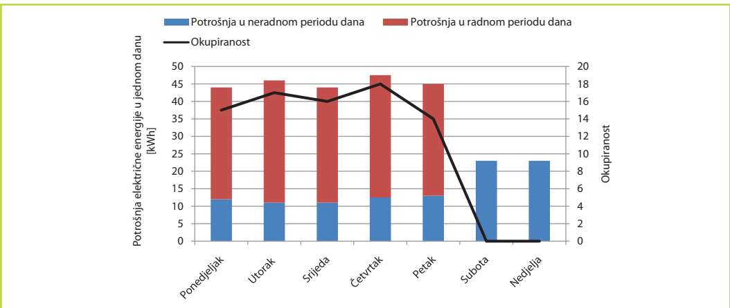
Slika 6-1: Primjer prikaza dnevne potrošnje električne energije po funkcijskim periodima i razine okupiranosti u odabranom tjednu
