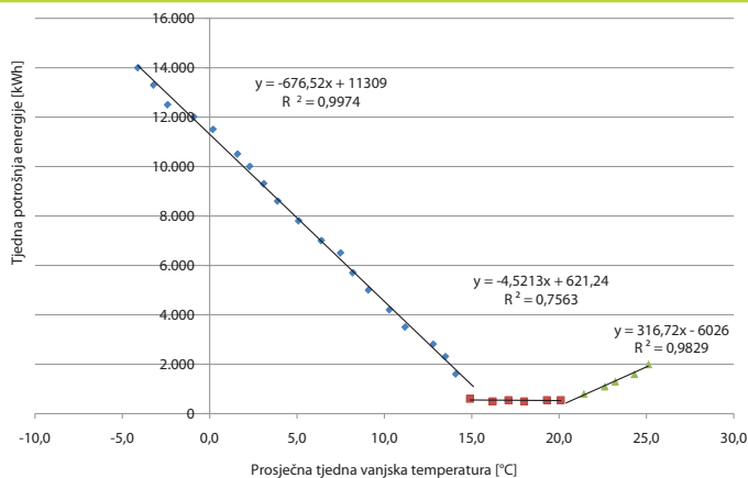
Slika P-6: Prikaz tjedne potrošnje energije u ovisnosti o vanjskoj temperaturi (pokazni primjer linearne regresije E-t krivulja)
