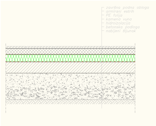
Slika 8. Izolirani pod
