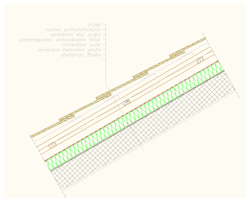
Slika 6. Izolirani krov
