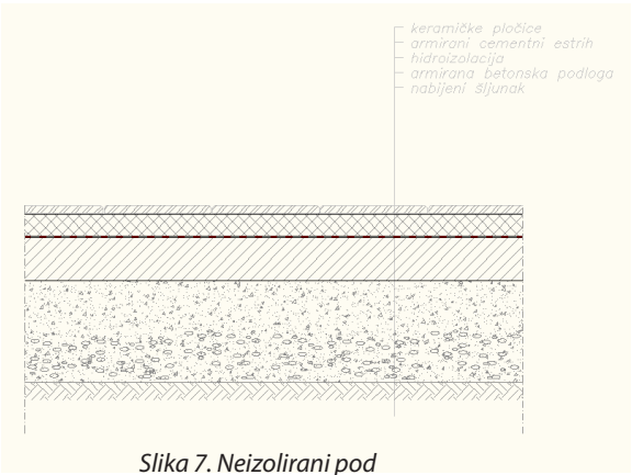
Slika 7. Neizolirani pod
