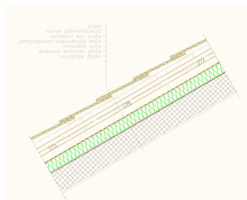
Slika 6. Izolirani krov
