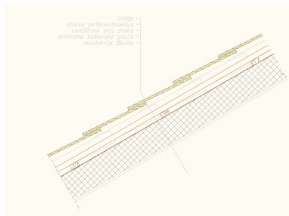
Slika 5. Neizolirani krov
