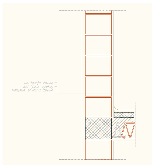
Slika 3. Neizolirani zid
